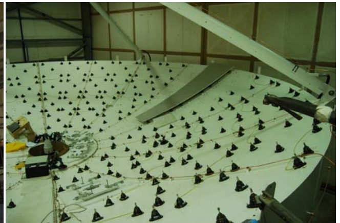
▲ 調整中のヨーロッパのアンテナ面
